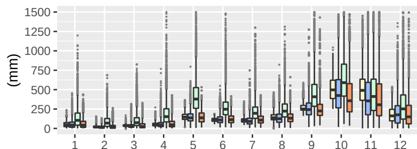
Reg6-clWRF-LT01
