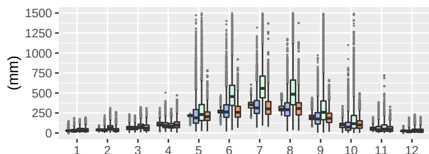
Reg3-clWRF-LT01
