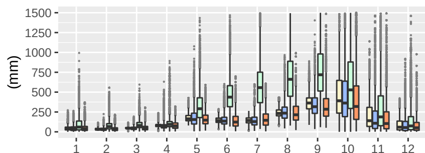
Reg5-clWRF-LT01
