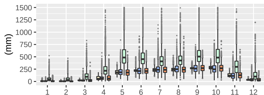
Reg7-clWRF-LT01
