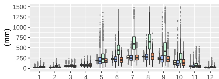
Reg4-clWRF-LT01
