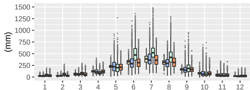
Reg2-clWRF-LT01
