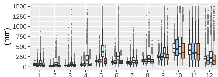
Reg6-clWRF-LT02
