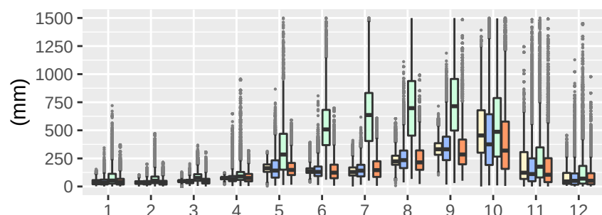
Reg5-clWRF-LT02
