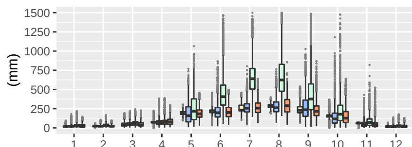
Reg4-clWRF-LT02
