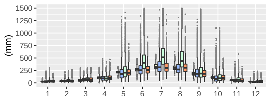
Reg3-clWRF-LT02
