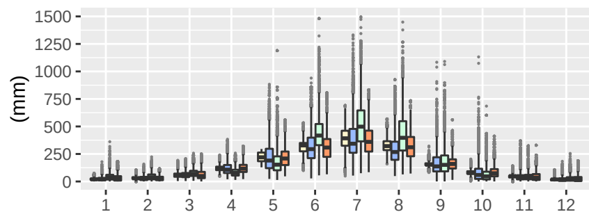
Reg2-clWRF-LT02
