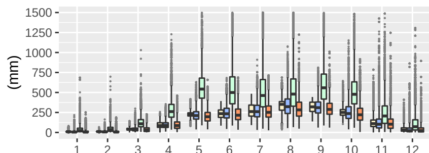
Reg7-clWRF-LT02
