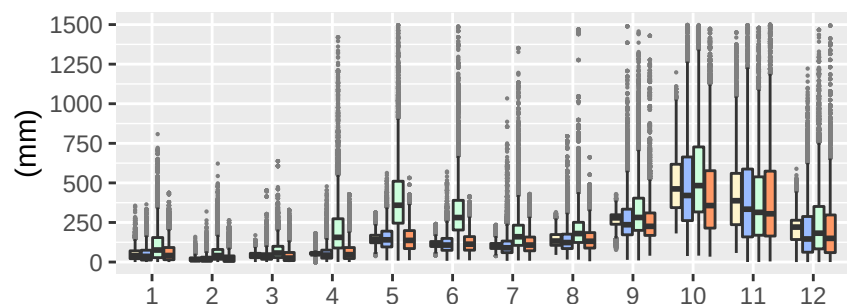
Reg6-clWRF-LT05
