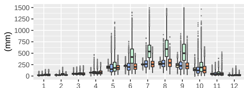
Reg4-clWRF-LT05
