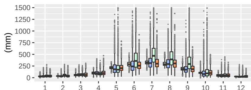
Reg3-clWRF-LT05
