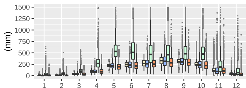
Reg7-clWRF-LT05
