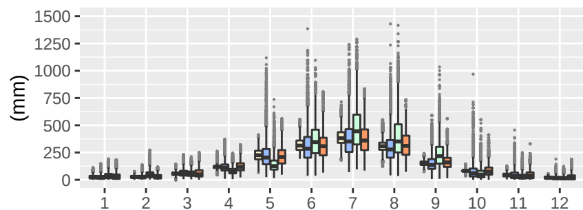
Reg2-clWRF-LT05
