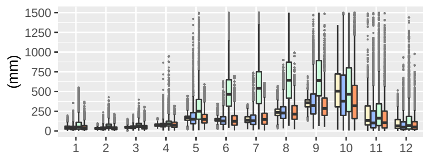
Reg5-clWRF-LT05
