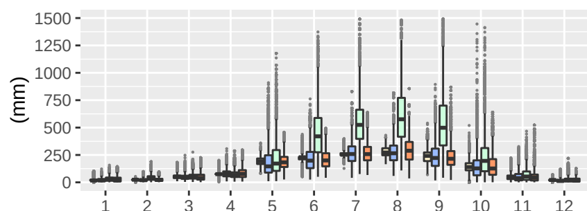
Reg4-clWRF-LT06
