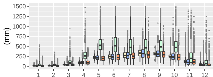
Reg7-clWRF-LT06
