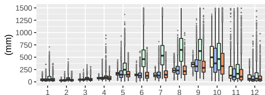
Reg5-clWRF-LT06
