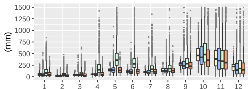
Reg6-clWRF-LT06
