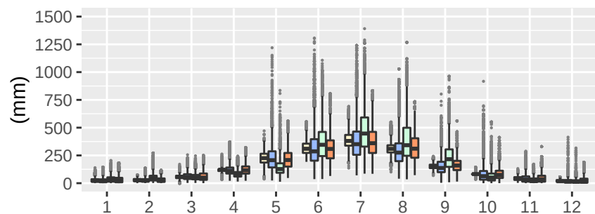
Reg2-clWRF-LT06
