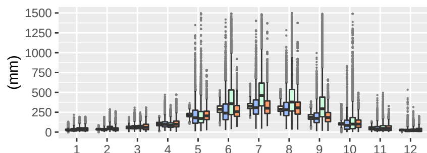
Reg3-clWRF-LT06
